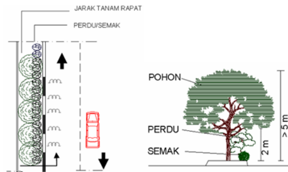
Gambar 2. Ilustrasi Perdam Kebisingan (Sumber: Permen no.5 2008)
