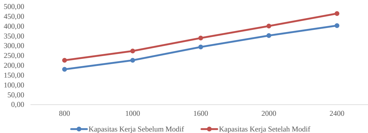
Gambar 2. Kapasitas kerja sebelum dan sesudah dimodifikasi
