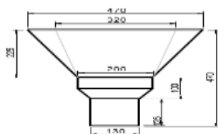
Hopper Input 40 derajat Sebelum Modifikasi
